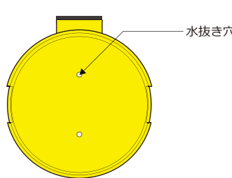
上面図
